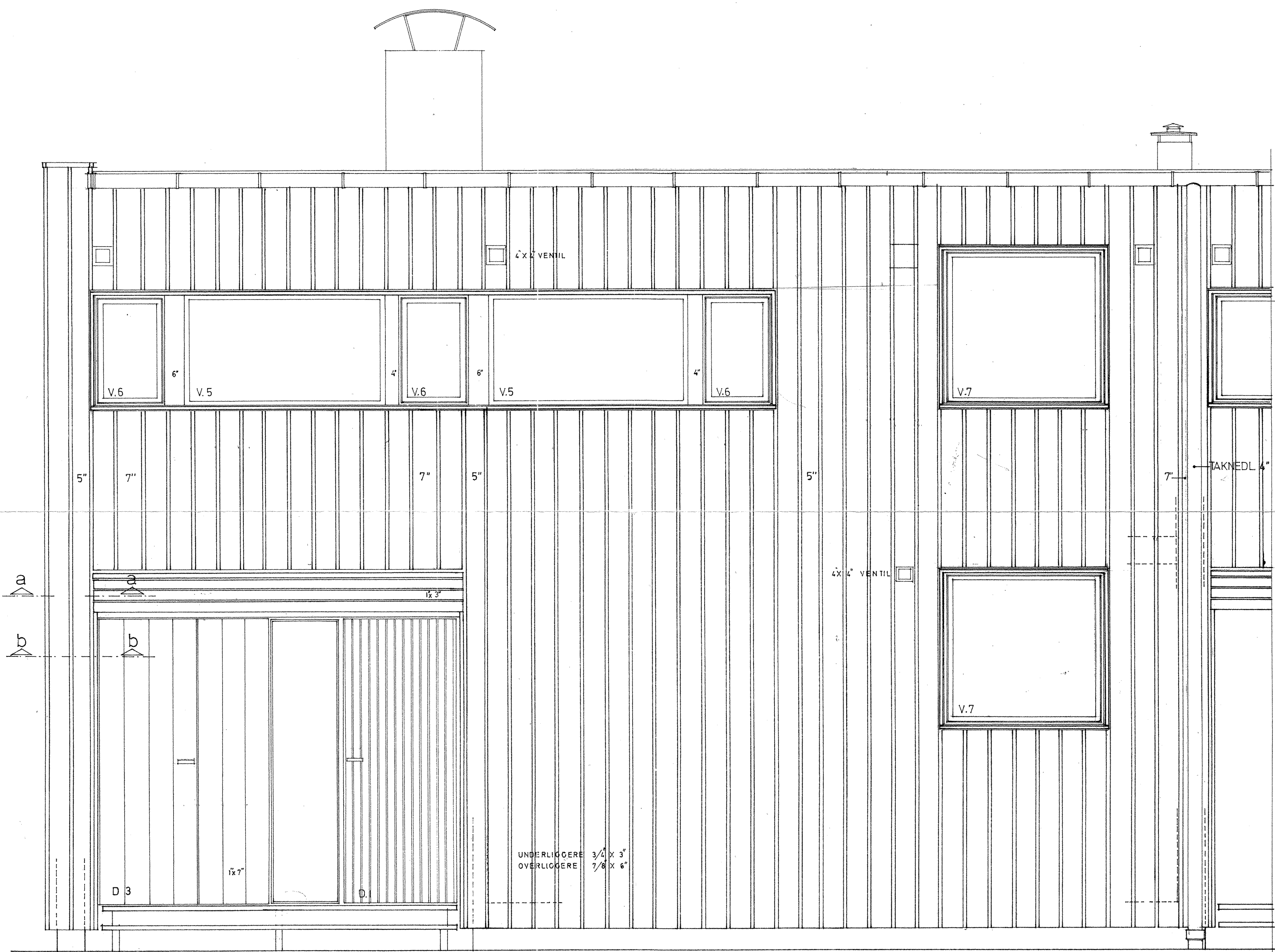
FASADE ÖST
