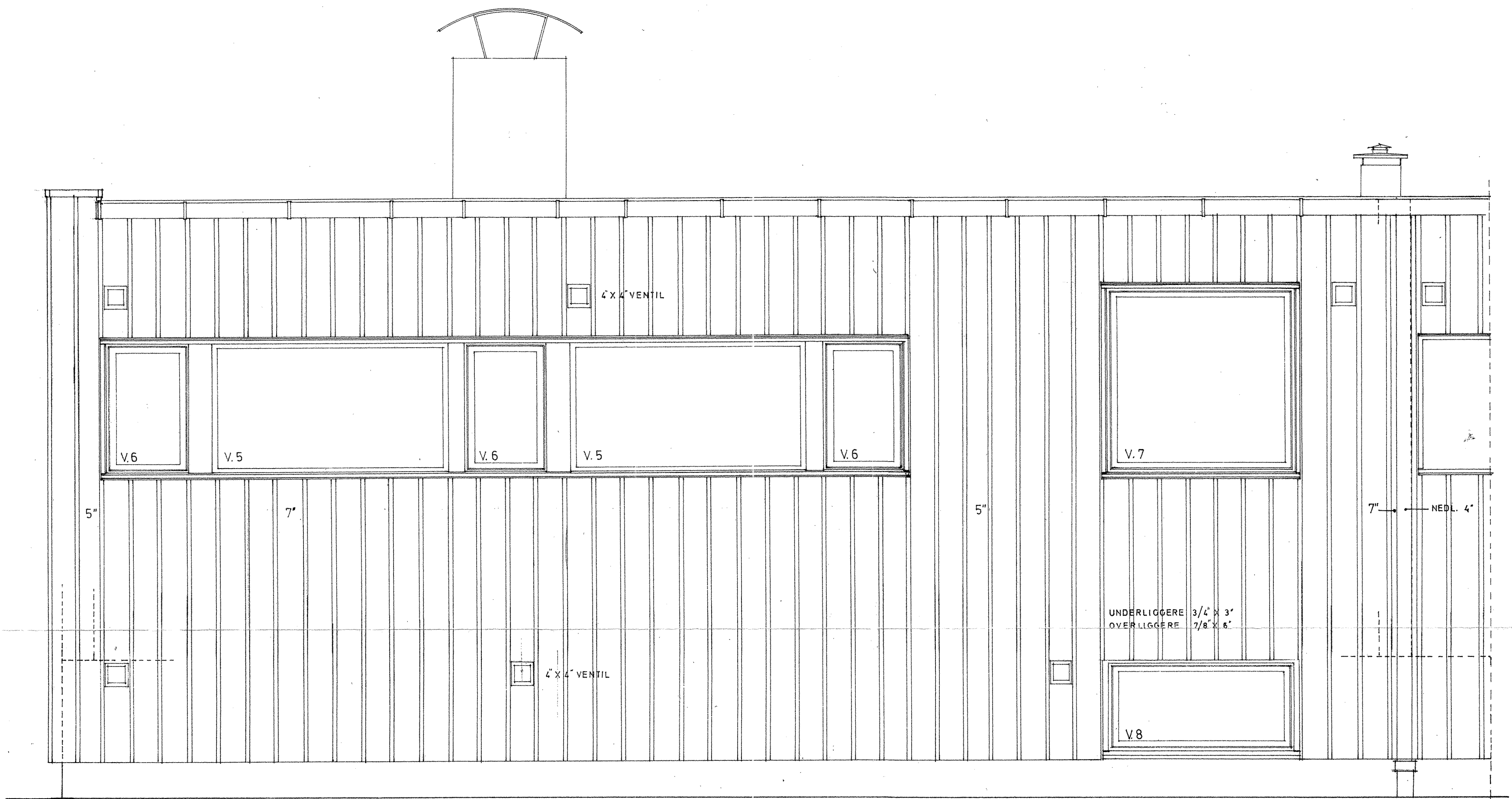
FASADE ÖST
