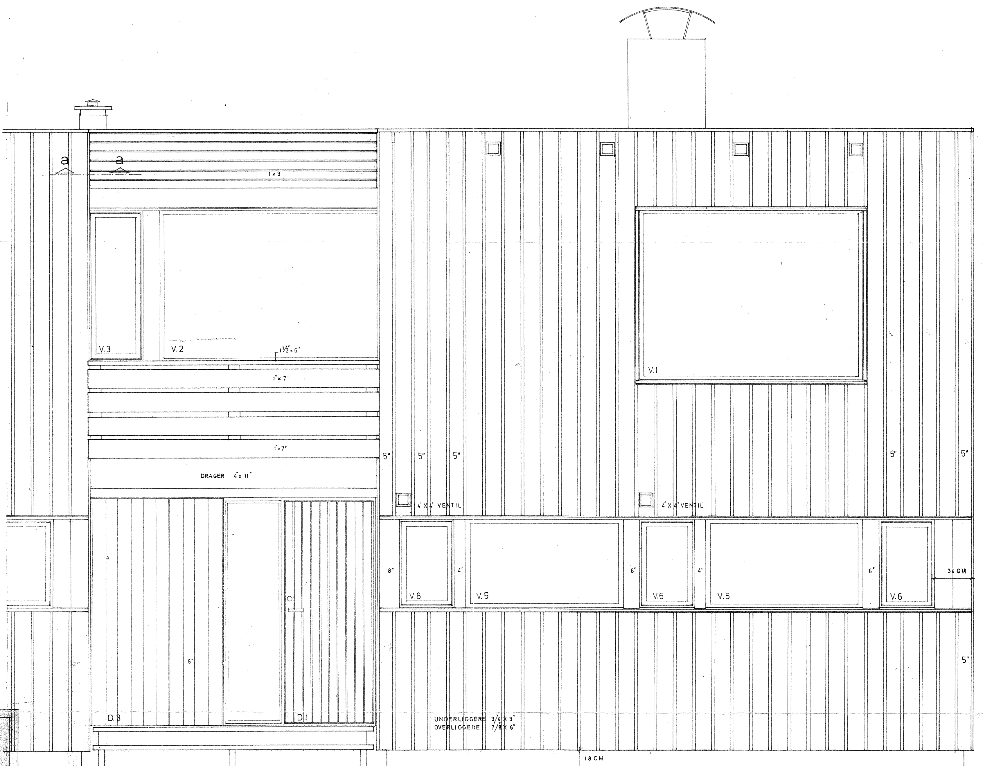
FASADE VEST
