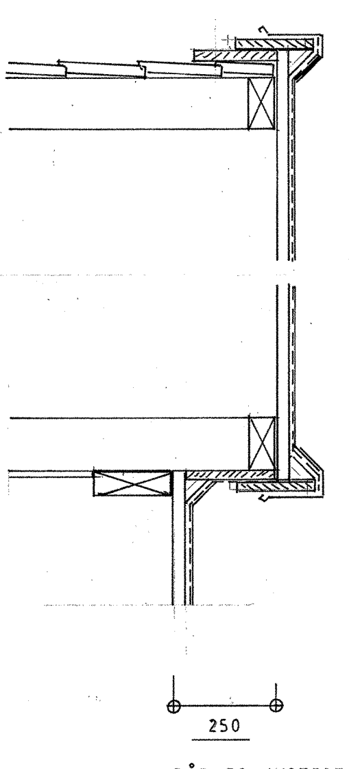
GAVL
